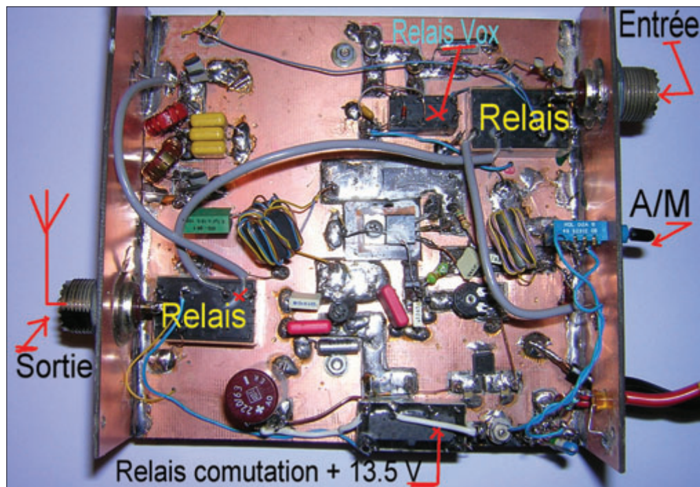
Photo 3 - Disposition des composants.
