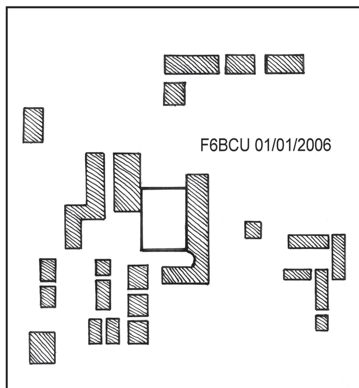
Figure 4 - Circuit imprimé L13 x H 14. Détail des pistes cuivre. Attention : le plan de masse existe, il reste blanc.
