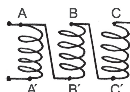
Figure 2 - Construction de TR1 et TR2.
