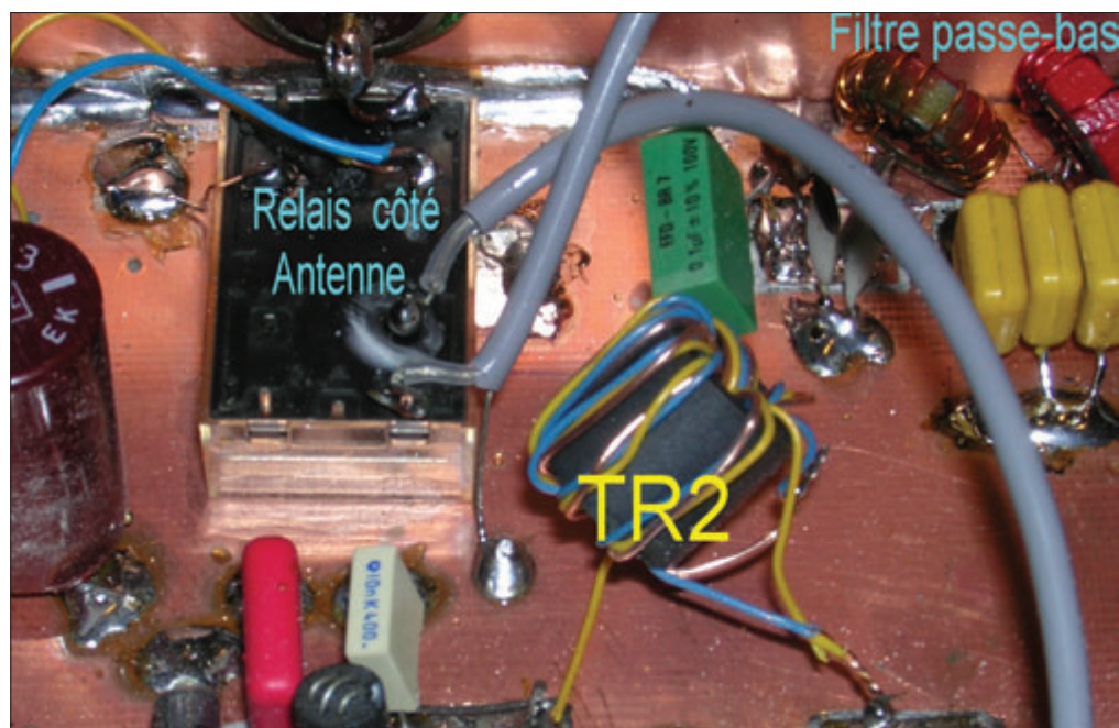
Photo 5 - Filtre passe-bas. Relais côté antenne. TR2.
