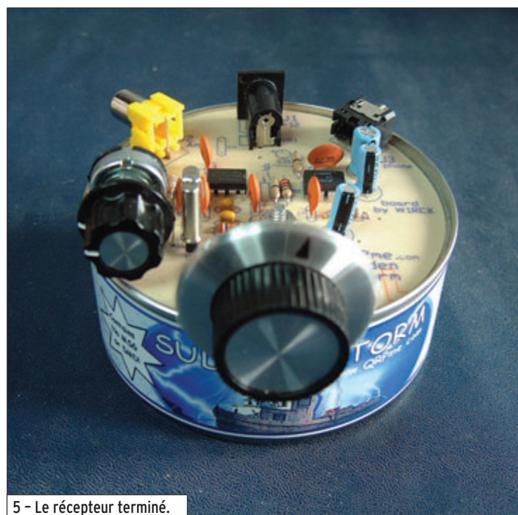
5 - Le récepteur terminé.
