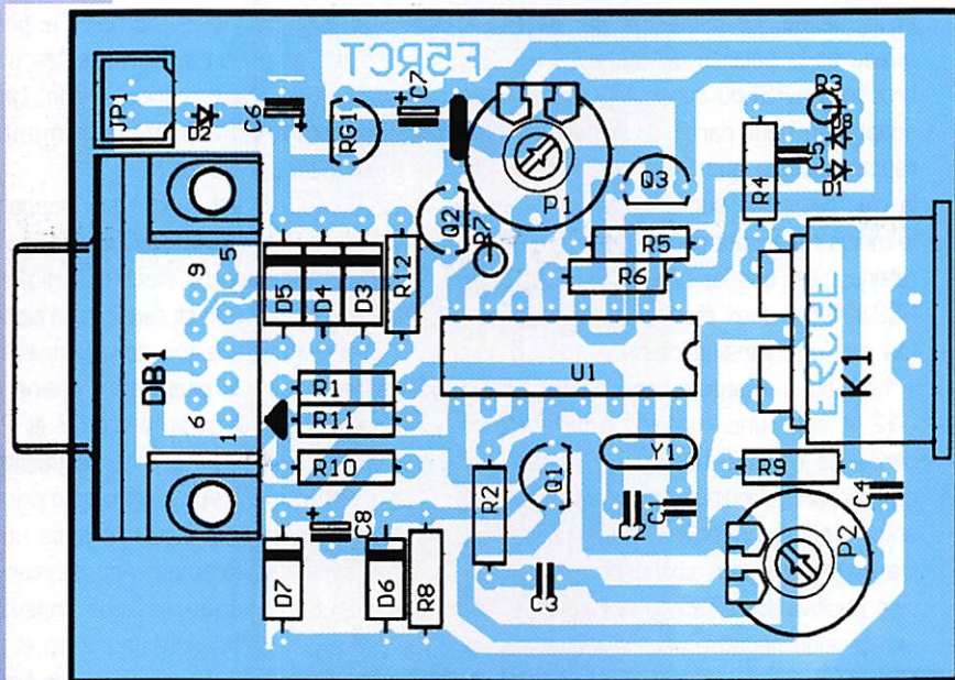
Implantation des composants.
